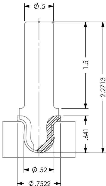
DISPOSABLE TOOL
