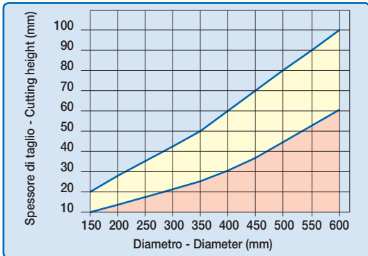
Altezza di taglio lungo e trasverso vena massima consentita in funzione del diametro della lama.
