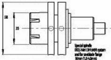
K1 ER25 Mini Nut DIN 6499
